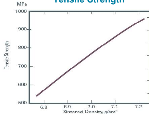
Tensile Strength
