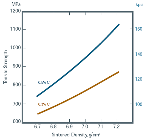
Tensile Strength
