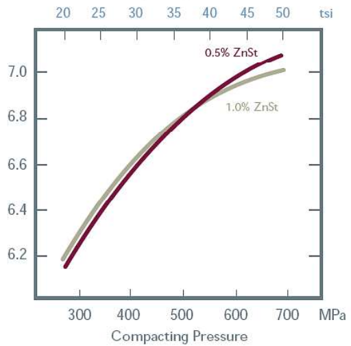
ATOMET 29 + ZnSt
